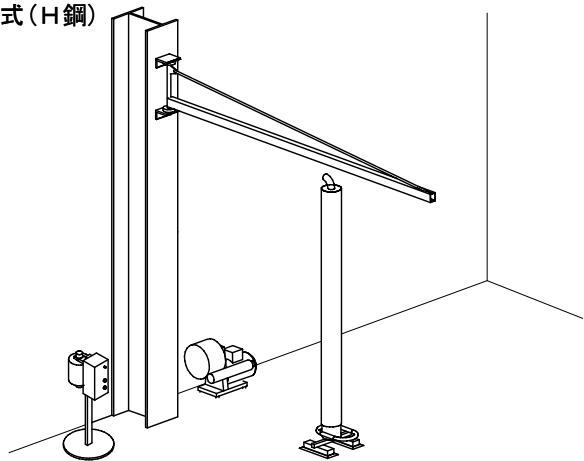
側柱固定式（H鋼）
