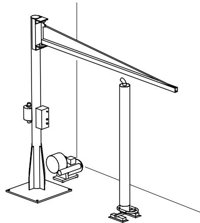
床上固定式架台
